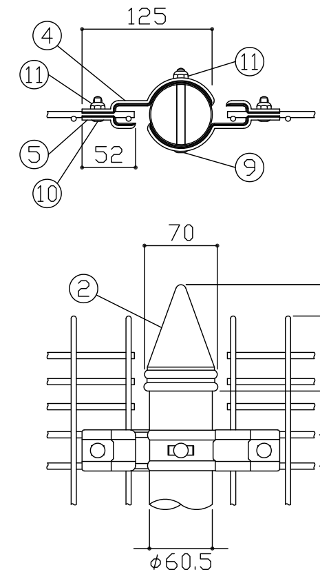
A部詳細図 S = 1 / 5
