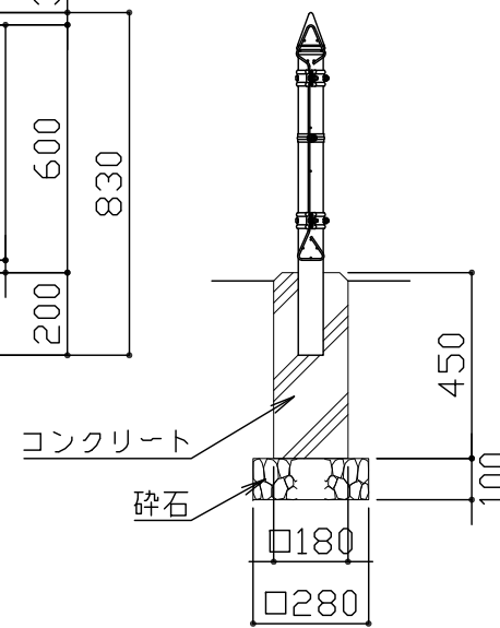
側面図 S = 1 / 20
