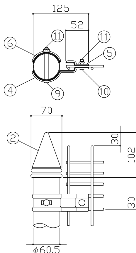
C部詳細図 S = 1 / 5
