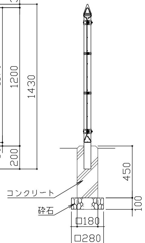
側面図 S = 1 / 20
