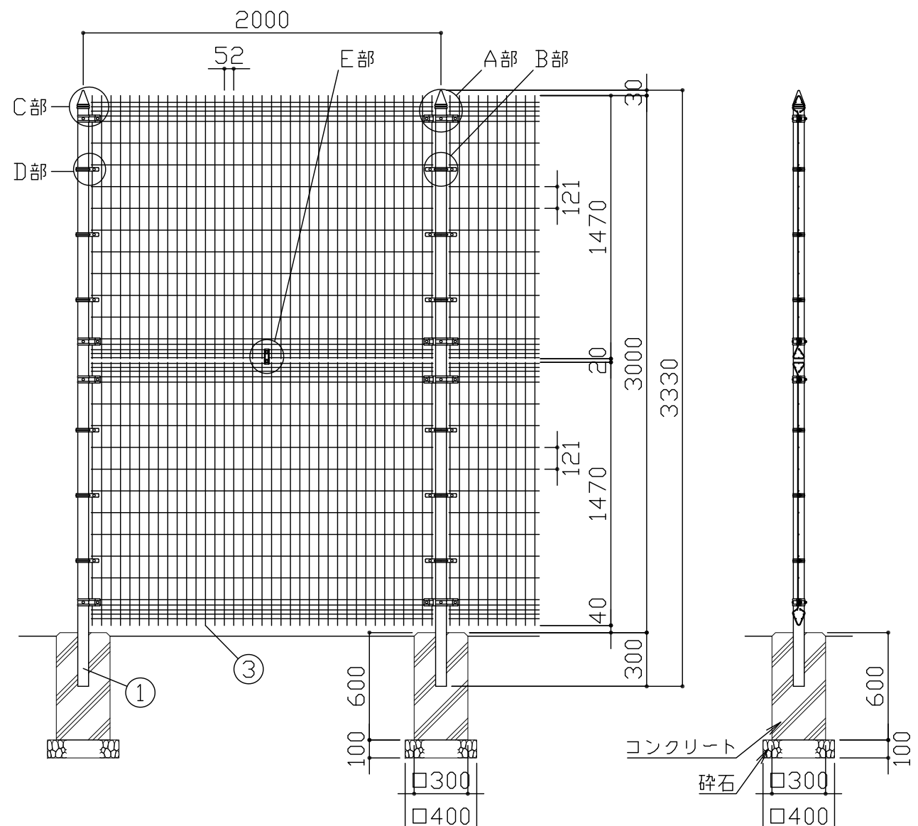
立面図 S = 1 / 30
