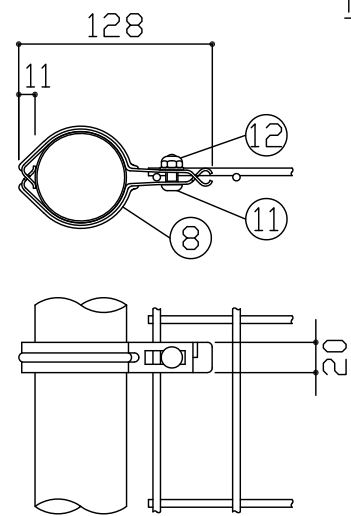
D部詳細図 S = 1 / 5
