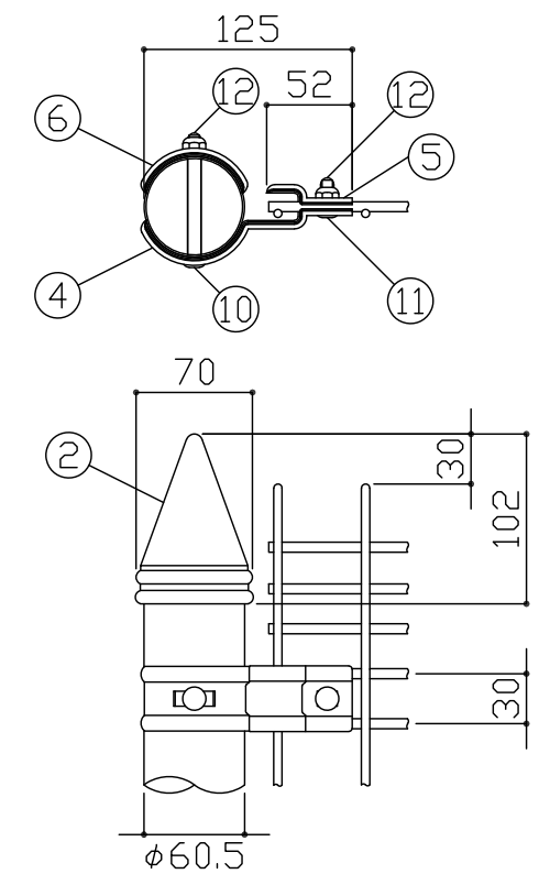
C部詳細図 S = 1 / 5
